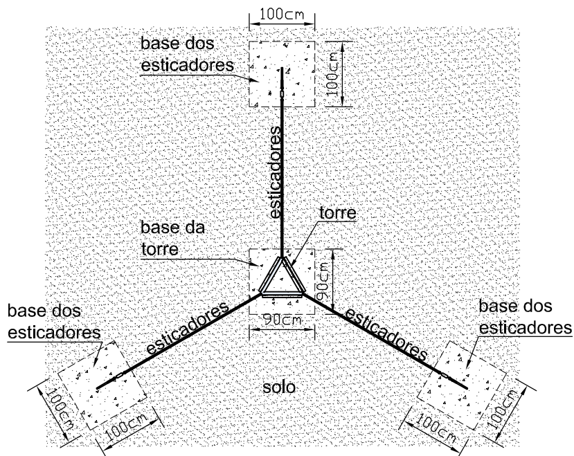
VISTA SUPERIOR
