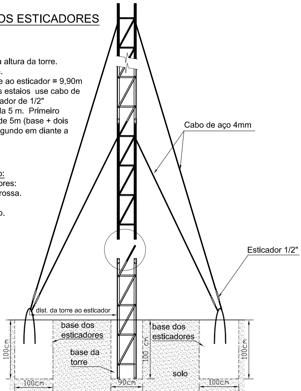
VISTA LATERAL
